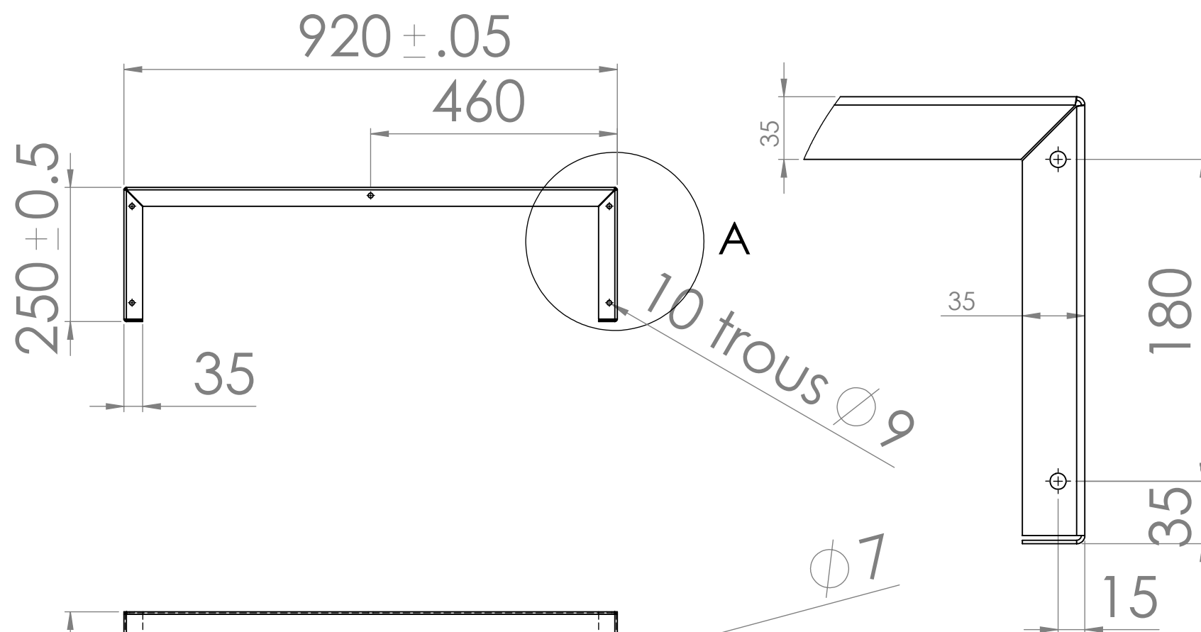
DÉTAIL A ECHELLE 1 : 3
